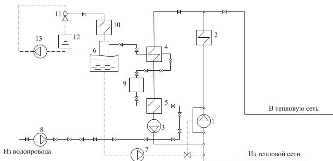
Рисунок 2.3 – Принципиальная тепловая схема котельной с водогрейными котлами:
