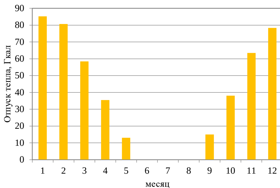
Рисунок 1.4 – Оптимальный температурный график отпуса тепловой энергии для Котельной «Школьная» с. Нарга
