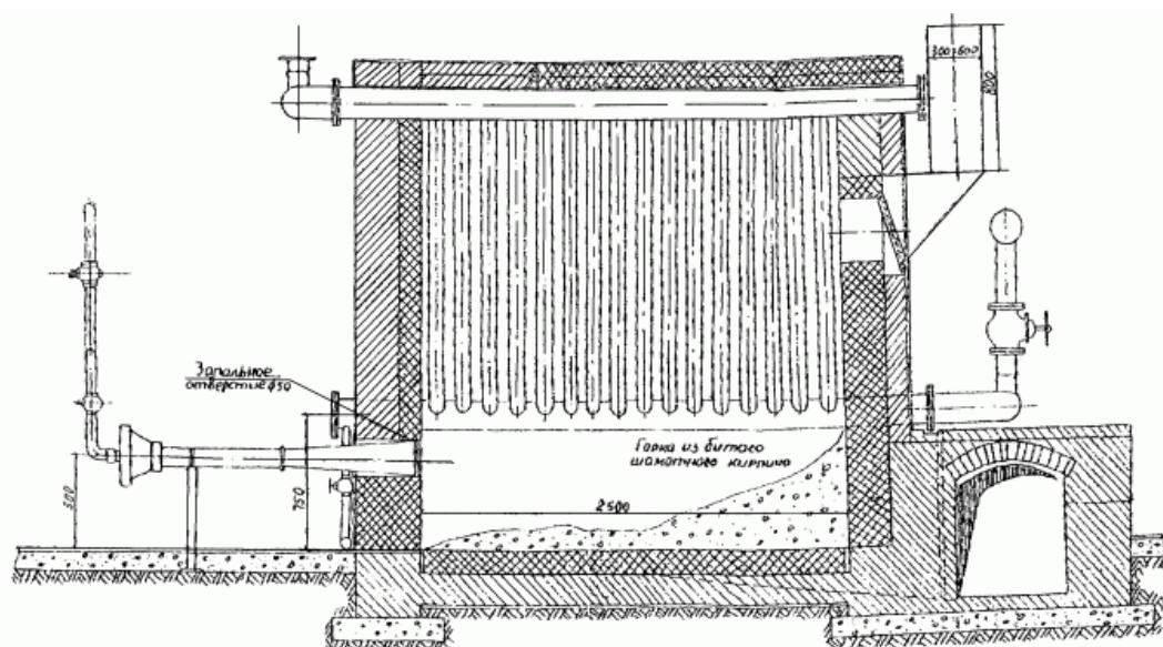
Рисунок 2.1 Схема котла "НР-18"
