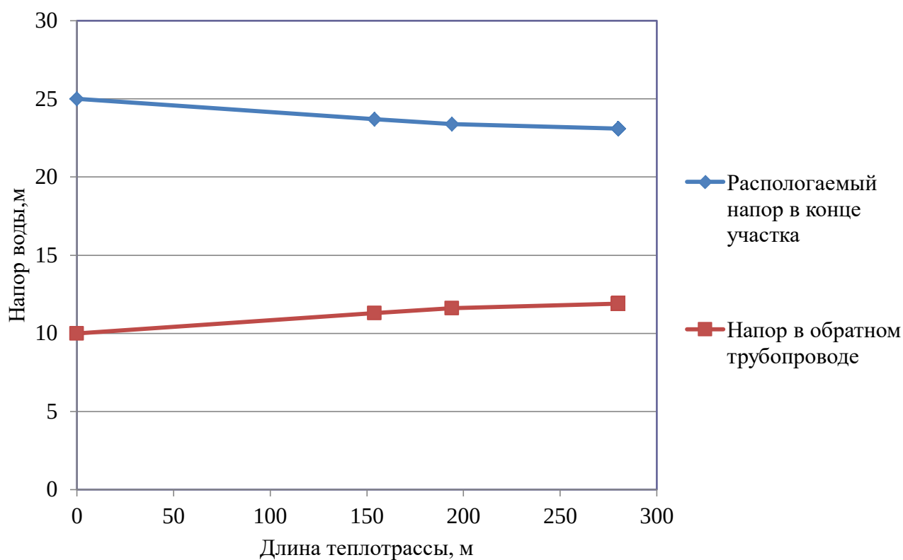
Рисунок 2.6 – Пьезометрический график тепловой сети Котельной «Школьная» с. Нарга
