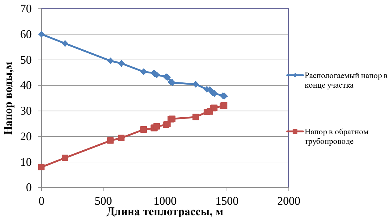
Рисунок 2.10 – Пьезометрический график тепловой сети Котельной «Поселковая» с. Нарга
