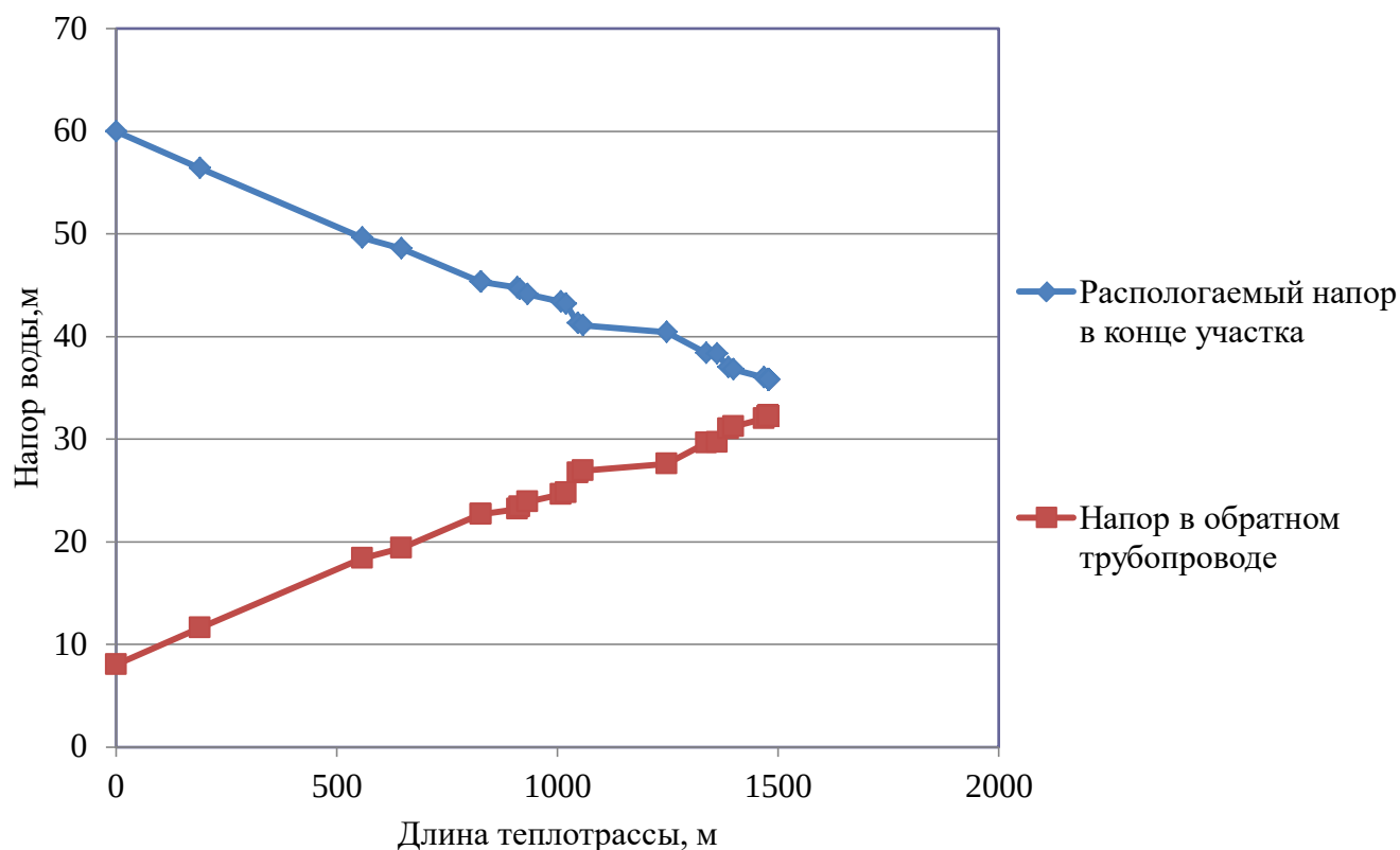
Рисунок 2.7 – Пьезометрический график тепловой сети Котельной «Поселковая» с. Нарга
