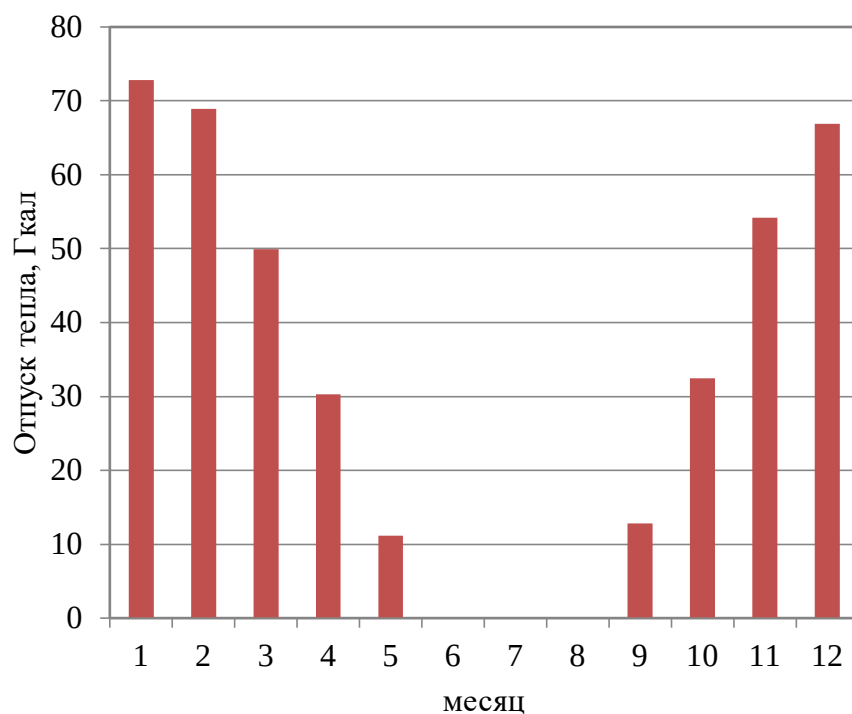
Рисунок 1.3 – Оптимальный температурный график отпуса тепловой энергии для котельной «Больничная» с. Нарга с температурным режимом 95-70 °С
