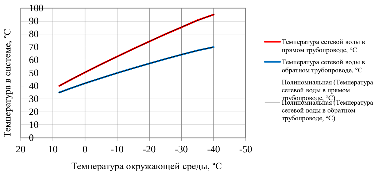
Рисунок 2.4– График изменения температур теплоносителя 95–70°C
