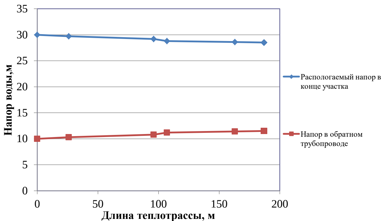
Рисунок 2.8 – Пьезометрический график тепловой сети Котельной «Больничная» с. Нарга
