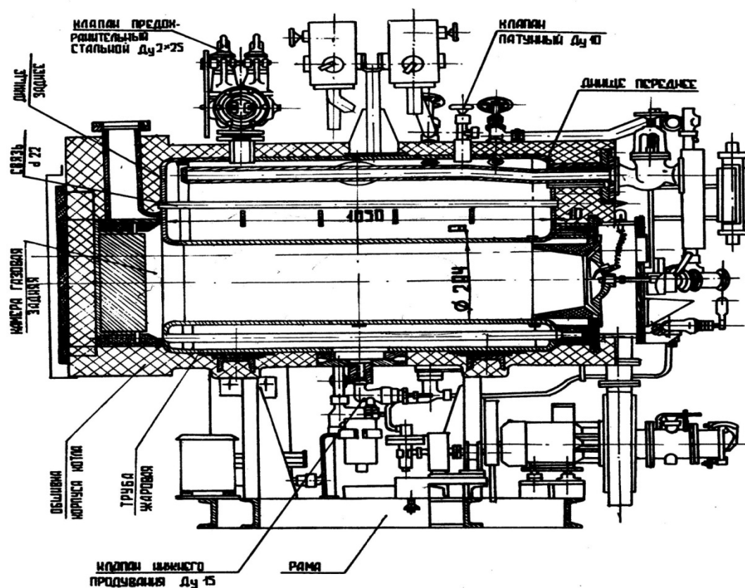
Рисунок 2.2 Схема котла «КВА 0,25Г-ЭЭ»
