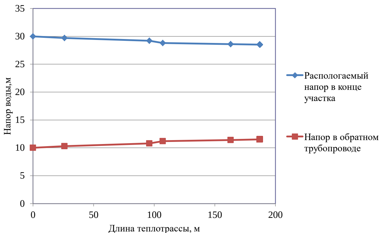
Рисунок 2.5 – Пьезометрический график тепловой сети Котельной «Больничная» с. Нарга
