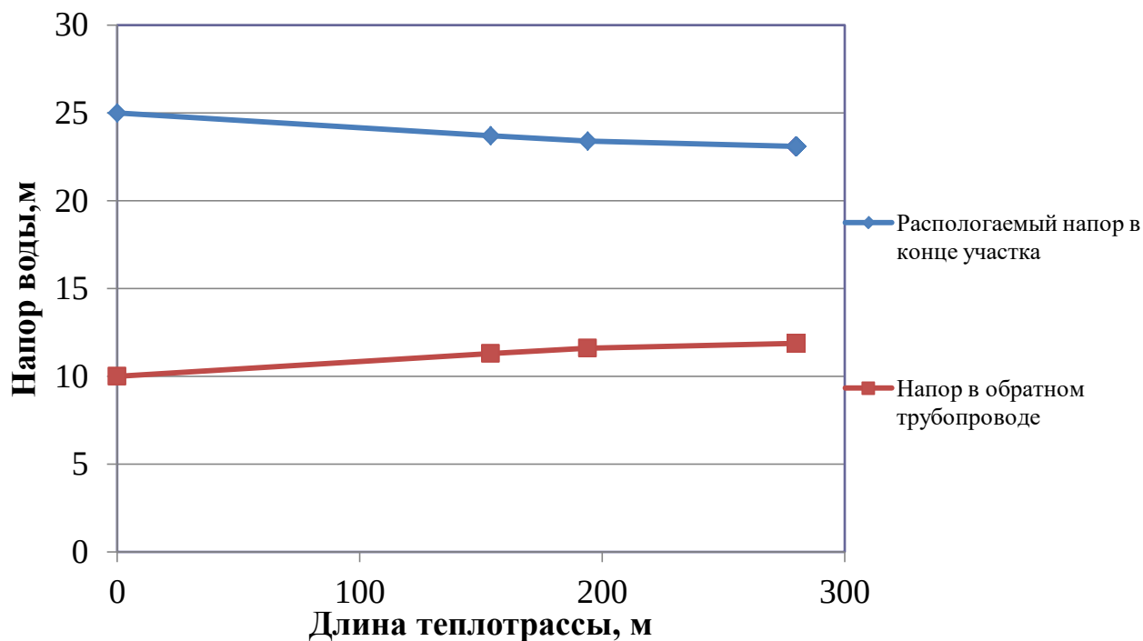
Рисунок 2.8 – Пьезометрический график тепловой сети Котельной «Больничная» с. Нарга
