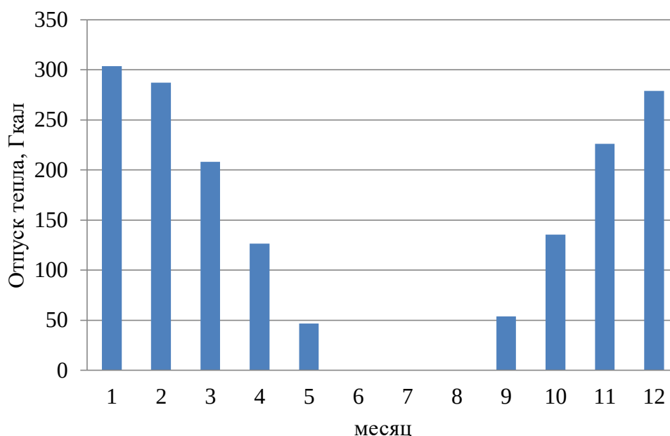
Рисунок 1.5 – Оптимальный температурный график отпуса тепловой энергии для котельной «Поселковая» с. Нарга
